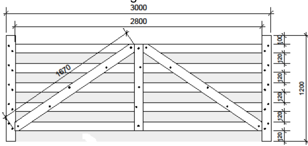
Eksempel på 3-meter bred grind (www.nsg.no)
